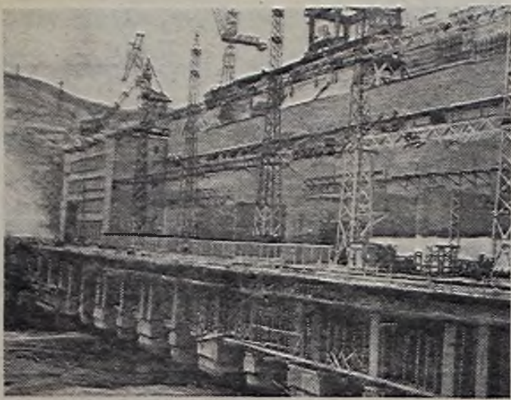
ВОСТОЧНО-КАЗАХСТАНСКАЯ ОБЛАСТЬ. Строители Бухартмaysкой ГЭС на укладке бетона достигли проектной отметки по всему фронту плотины и шитовой стенки. Четыре действующих агрегата с начала пуска ГЭС дали предприятиям Восточного Казахстана около 600 миллионов киловатт-часов дешевой электроэнергии. До конца третьего года семилетки будут сданы
