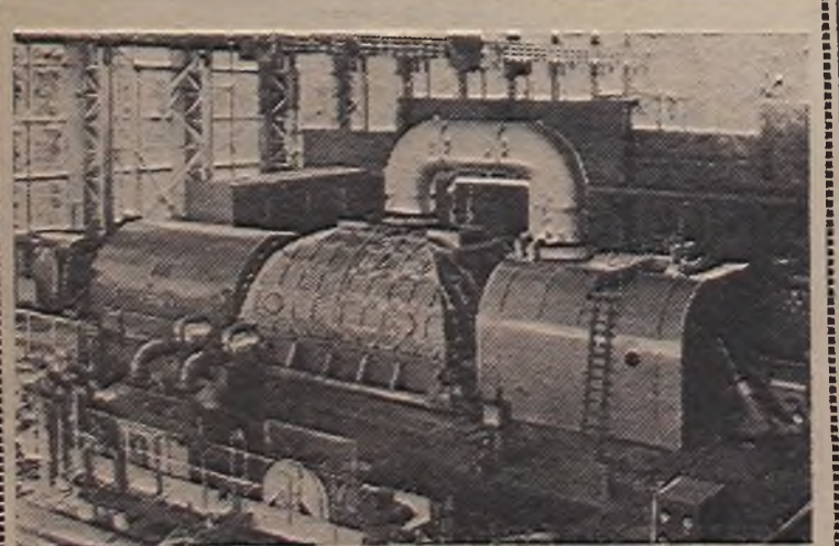
Красноярский край. Первый агрегат Назаровской ГРЭС дал промышленный ток и вступил в строй действующих. На снимке: турбогенератор № 1 Назаровской ГРЭС мощностью 150 тысяч киловатт. Фото Ю. Бармина. Фотохроника ТАСС.
